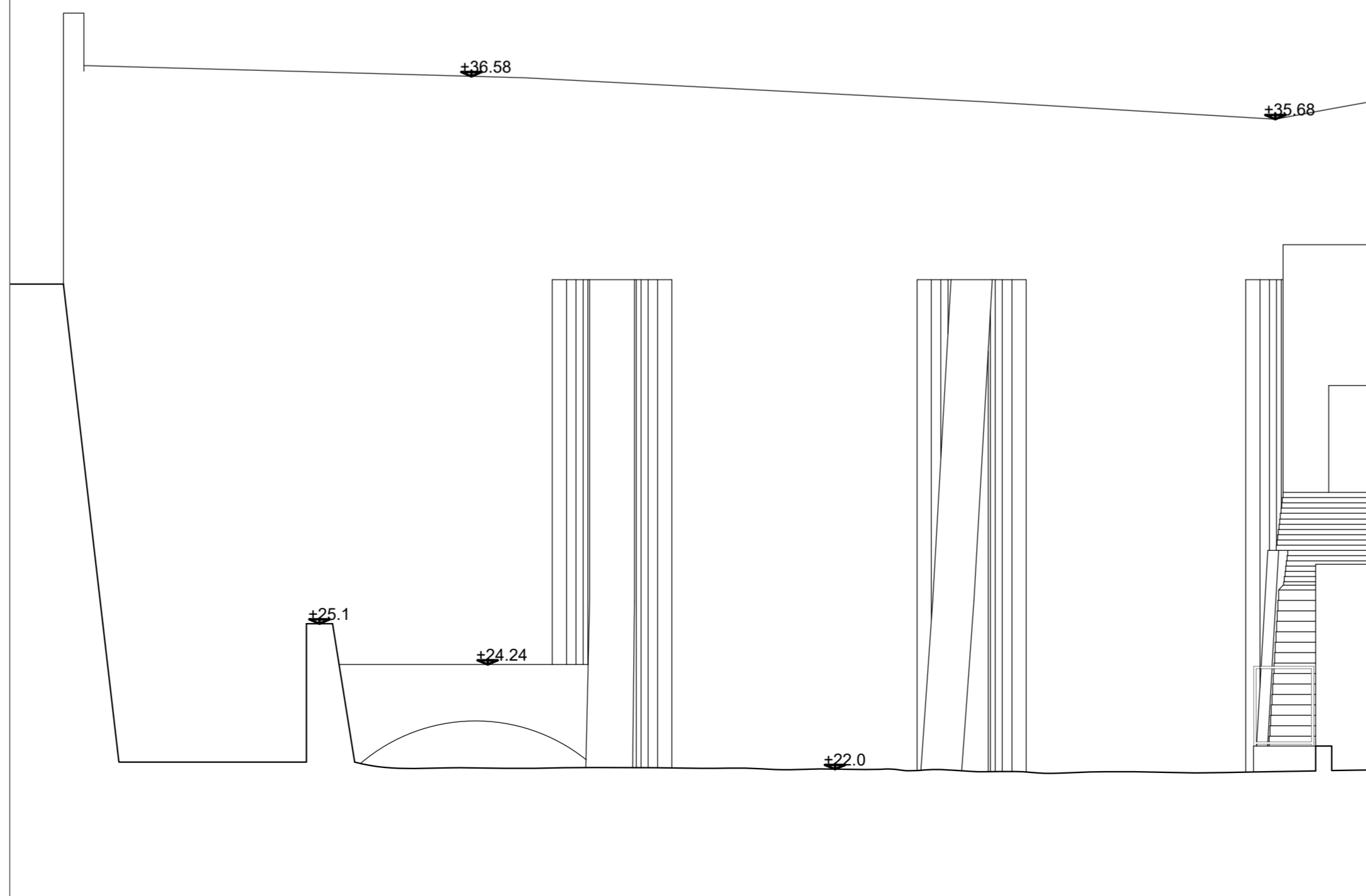
SEZIONE 7 SCALA 1:100
