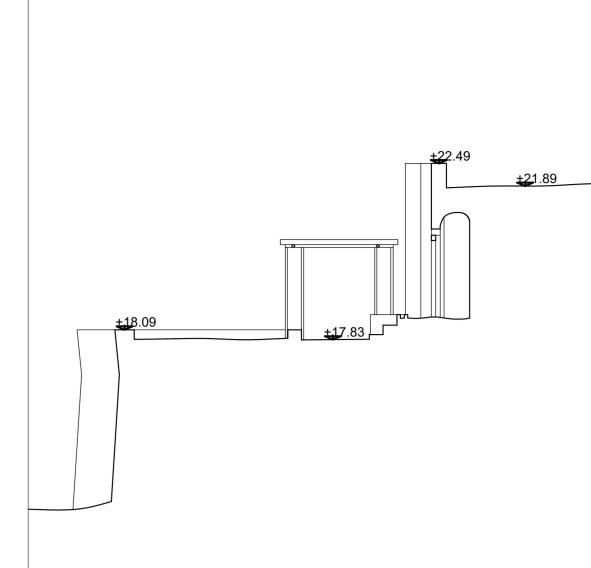
SEZIONE 17 SCALA 1:100
