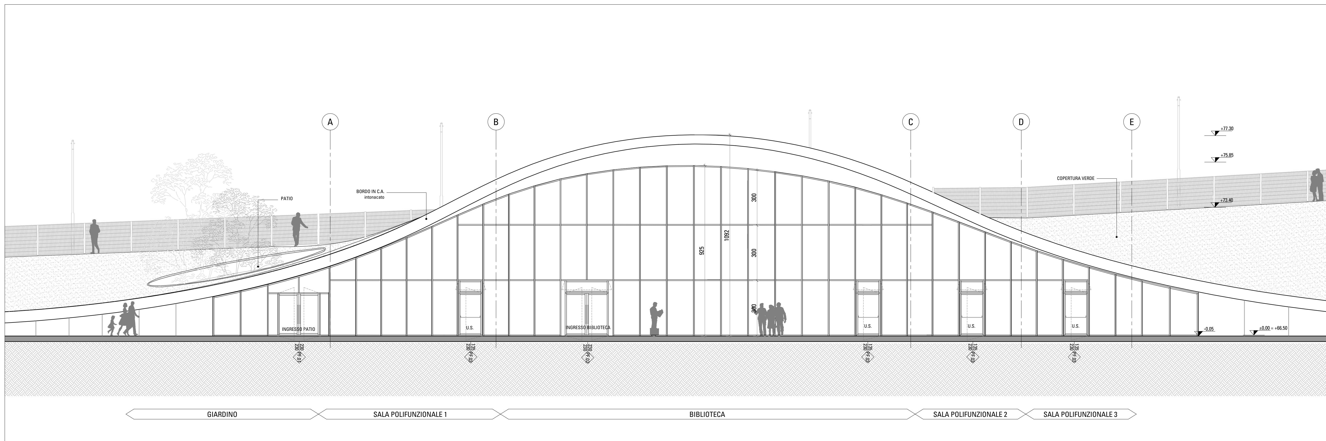
RES_E_PP 02 PROSPETTO OVEST Scala 1:100
